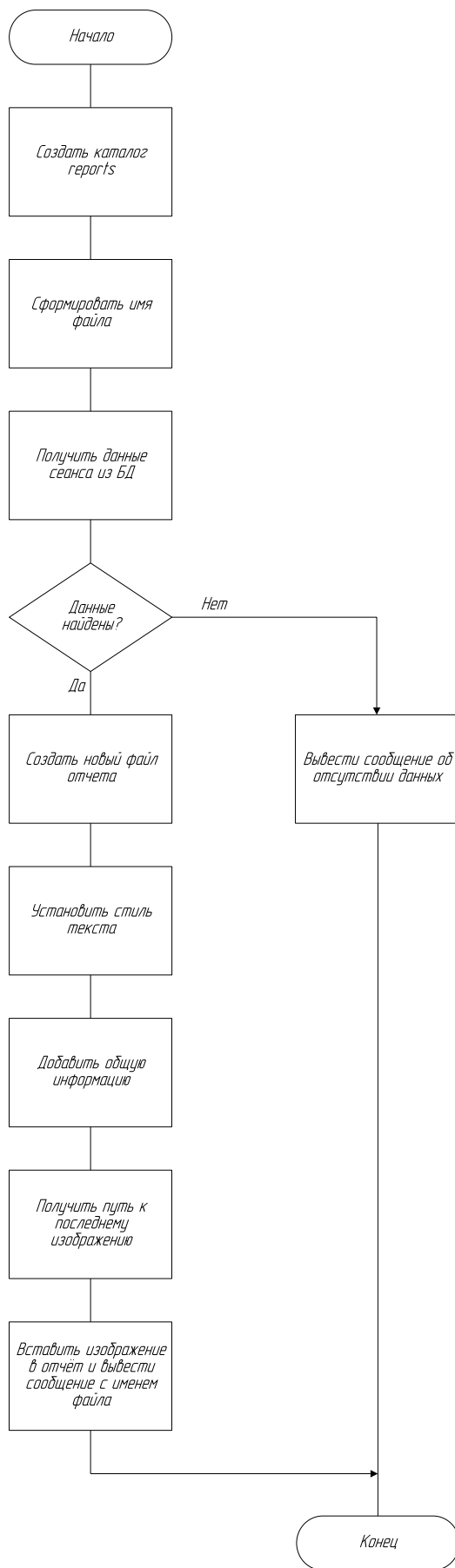
Рисунок 3.3 – Блок-схема алгоритма экспорта в файл в формате DOCX
