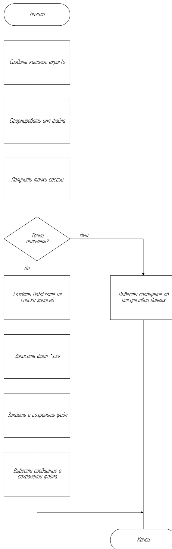
Рисунок 3.2 – Блок-схема алгоритма экспорта в файл в формате CSV
