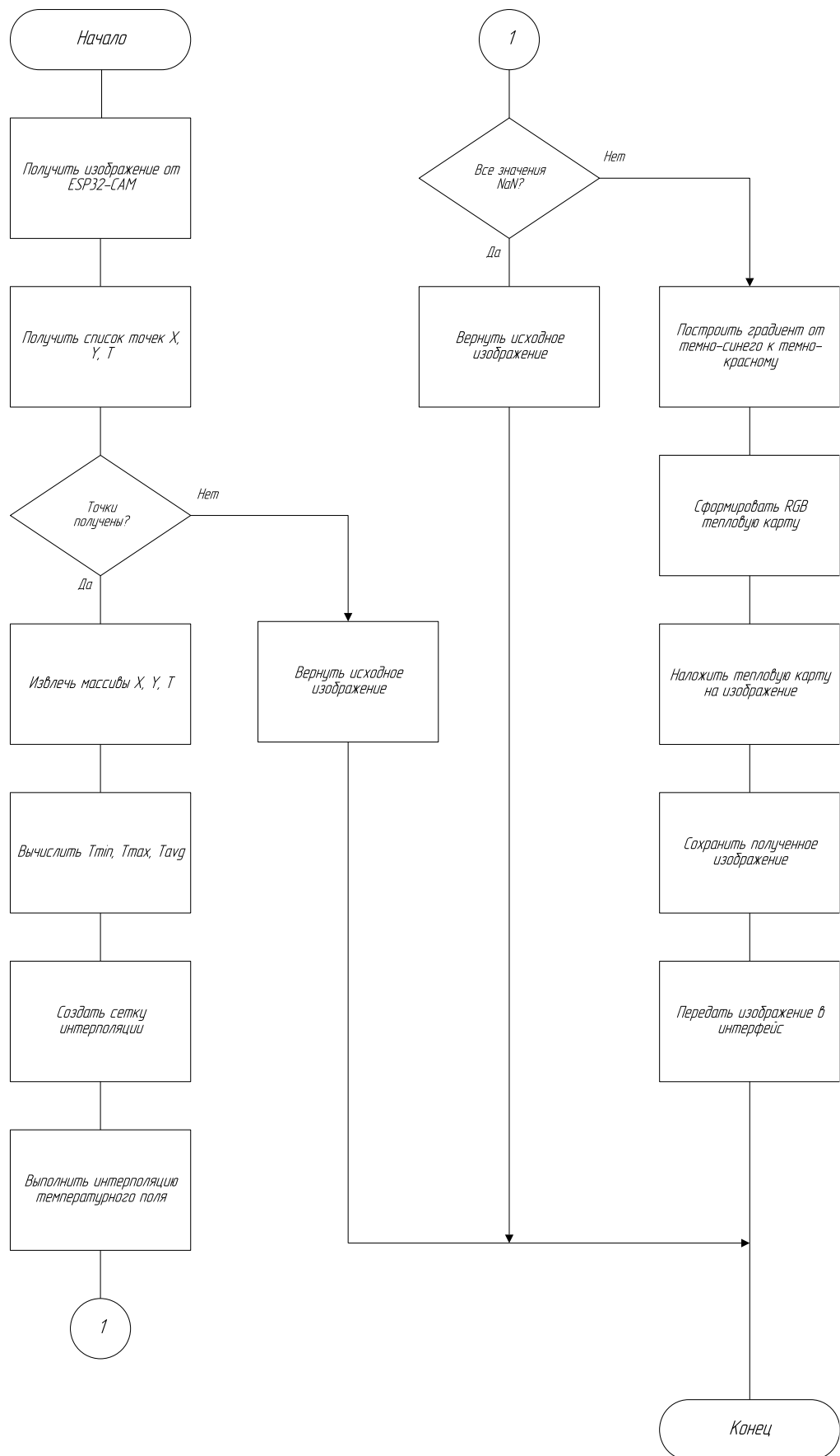
Рисунок 3.1 – Блок-схема алгоритма наложения температурной информации на изображение и сохранения в базу данных
